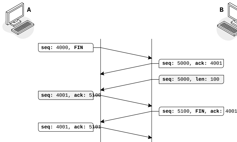
FIGURA 12.3: TCP: Patrón de mensajes de la desconexión en 4 segmentos
